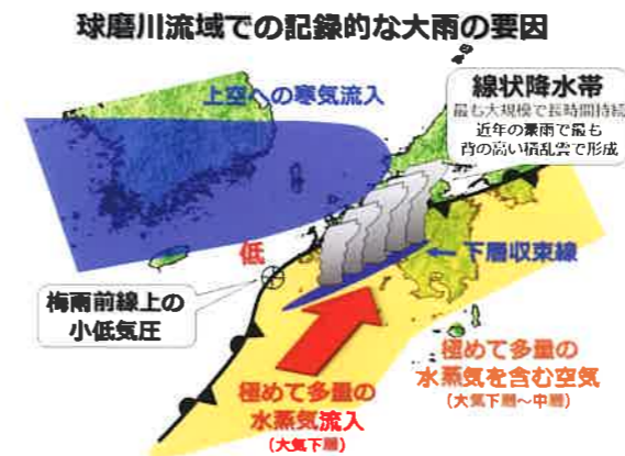
図 7月3~4日の球磨川流域における記録的な大雨の要因の概念図。 気象研究所報道発表資料より
